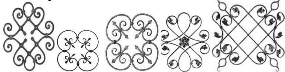
Nr 13.019 □ 12 mm H 460 mm L 410 mm Nr 13.020 10x5 mm H 380 mm L 380 mm Nr 13.025 □ 12 mm H 590 mm L 590 mm Nr 13.026 16x8 mm H 590 mm L 510 mm Nr 13.027 16x8 mm H 670 mm L 640 mm
