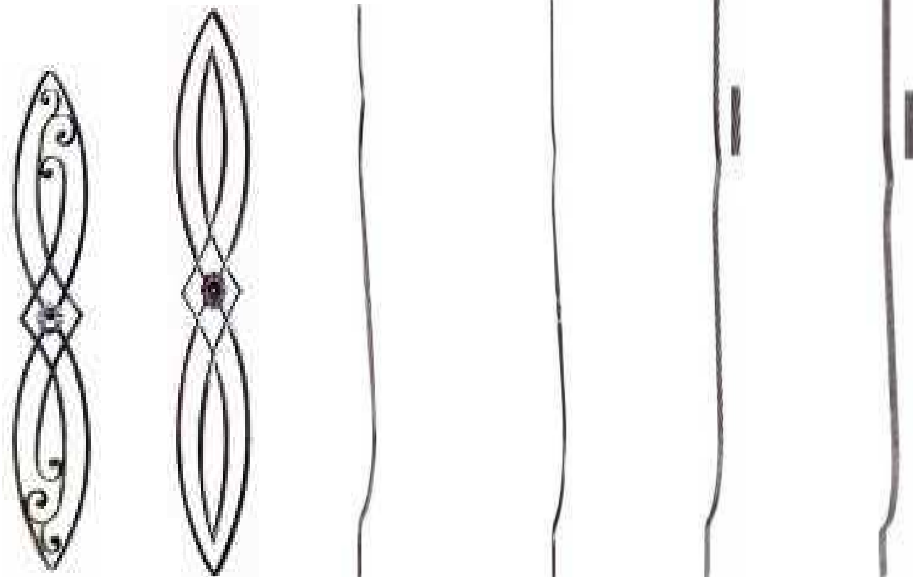
13.053 14x8 mm H 1 000 mm L 190 mm 13.054 14x8 mm H 1 000 mm L 190 mm 20.120 □ 12 mm H 1 000 mm 20.102 □ 12 mm H 1 000 mm 20.126 □ 32x5 mm H 1 000 mm 20.127 □ 31x5 mm H 1 000 mm
