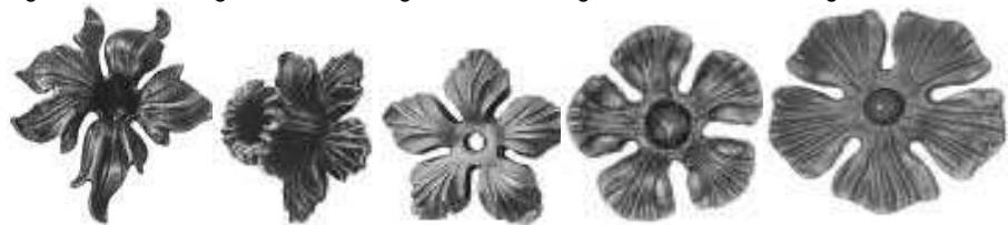
Nr 52.130 Nr 52.131 Nr 52.132 Nr 52.133 Nr 52.134 H 160 mm H 60 mm Otwór 8 mm Ø 90 mm Ø 90 mm L 160 mm Ø 90 mm Ø 90 mm Ø 90 mm Ø 90 mm grubość 4 mm grubość 3 mm grubość 3 mm grubość 5 mm grubość 5 mm
