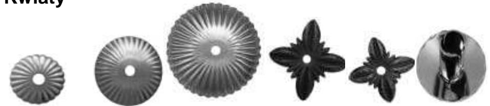
Nr 50.029 Nr 50.030 Nr 50.031 Nr 50.032 Nr 50.033 50.034 H 5 mm H 10 mm H 20 mm H 200 mm H 45 mm Ø 46 mm Ø 70 mm Ø 115 mm Ø 80 mm Ø 60 mm Ø 75 grubość 1,5 mm grubość 1,5 mm grubość 1,5 mm grubość 1,5 mm
