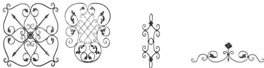
Nr 13.028 16x8 mm H 800 mm L 800 mm Nr 13.029 16x8 mm H 800 mm L 700 mm Nr 13.030 □ 12 mm H 900 mm L 385 mm Nr 13.031 12x6 mm H 230 mm L 740 mm
