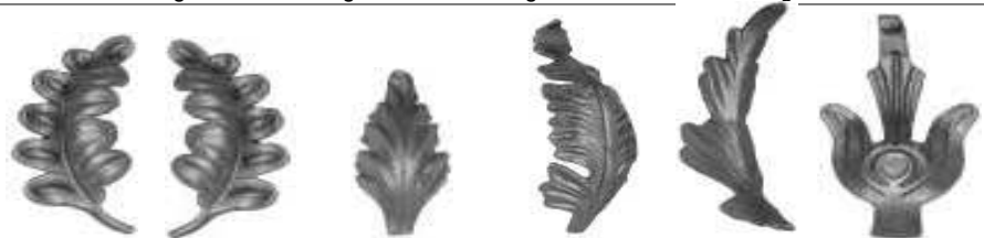
Nr 52.041 Nr 52.042 Nr 52.043 Nr 52.044 Nr 52.045 Nr 52.046 H 150 mm H 150 mm H 115 mm H 190 mm H 175mm H 155 mm L 55 mm L 55 mm L 55 mm L 60 mm L 50 mm L 90 mm grubość 4 mm grubość 4 mm grubość 4 mm grubość 4 mm grubość 4 mm grubość 4 mm
