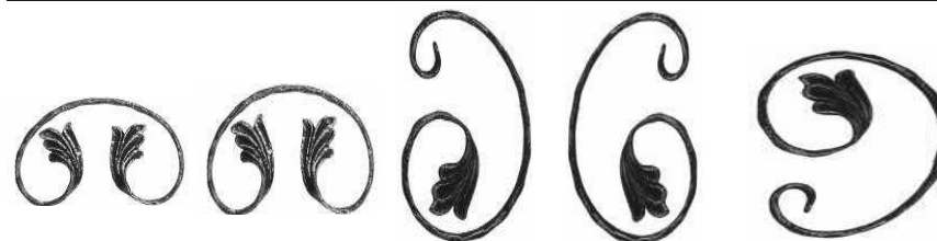
Nr 10.230 Nr 10.231 Nr 10.240 Nr 10.241 Nr 10.242 H 180 mm H 220 mm H 150 mm H 150 mm H 190 mm L 90 mm L 120 mm L 100 mm L 100 mm L 140 mm
