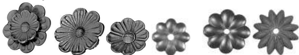
Nr 50.001 Nr 50.003 Nr 50.004 Nr 50.005 Nr 50.006 50.007 Ø 95 mm Ø 95 mm Ø 62 mm Ø 60 mm 90 Ø98 otwór 10 mm 10 12 grubość 5 mm grubość 5 mm grubość 4 mm grubość 3 mm grubość 3 mm
